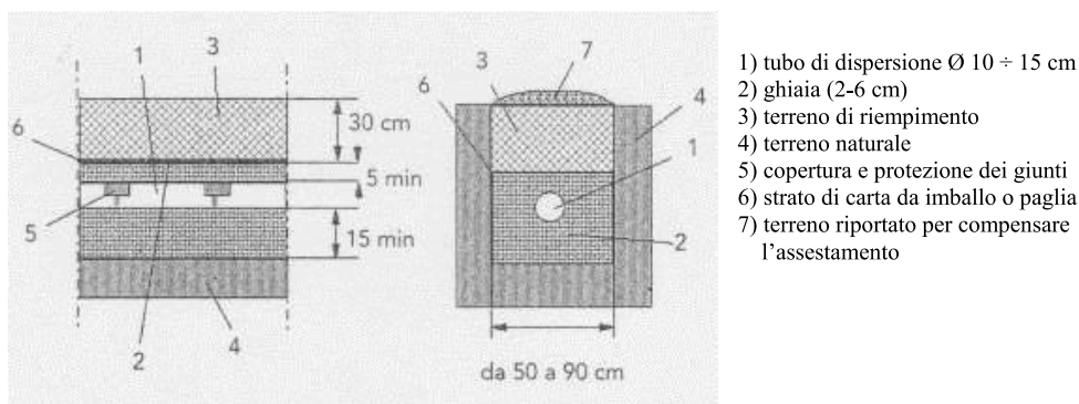
Figura 3.4 – Trincea drenante per la subdispersione nel terreno.
