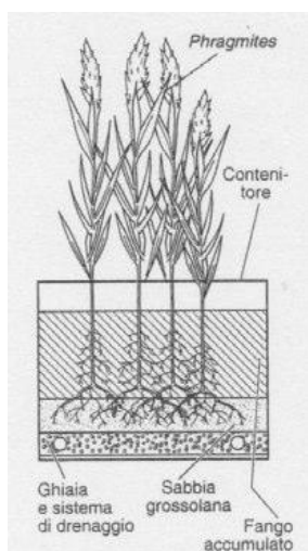
Figura 3.25 – Schema di fitodisidratazione.
