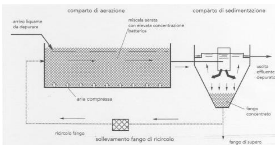
Figura 3.10 – Schema del processo a fanghi attivi.
