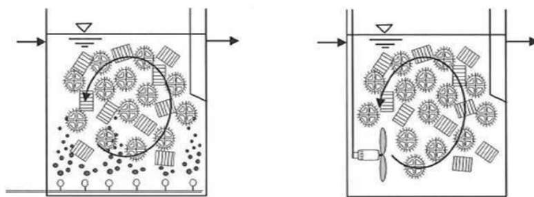
Figura 3.13 – Schema di un processo MBBR.
