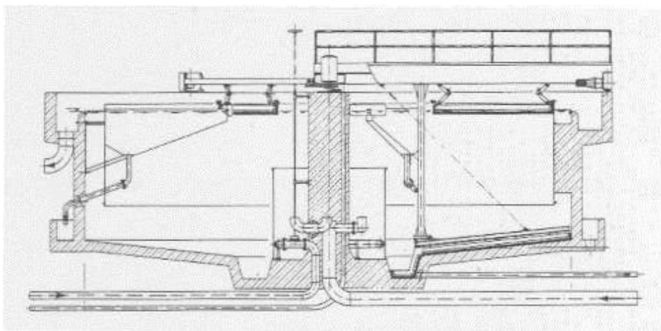
Figura 3.7 – Flottatore circolare.
