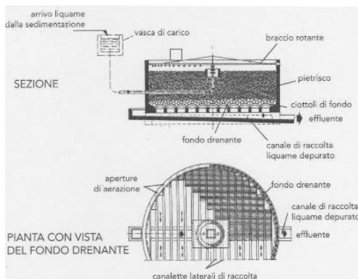
Figura 3.14 – Schema di un tradizionale letto percolatore.
