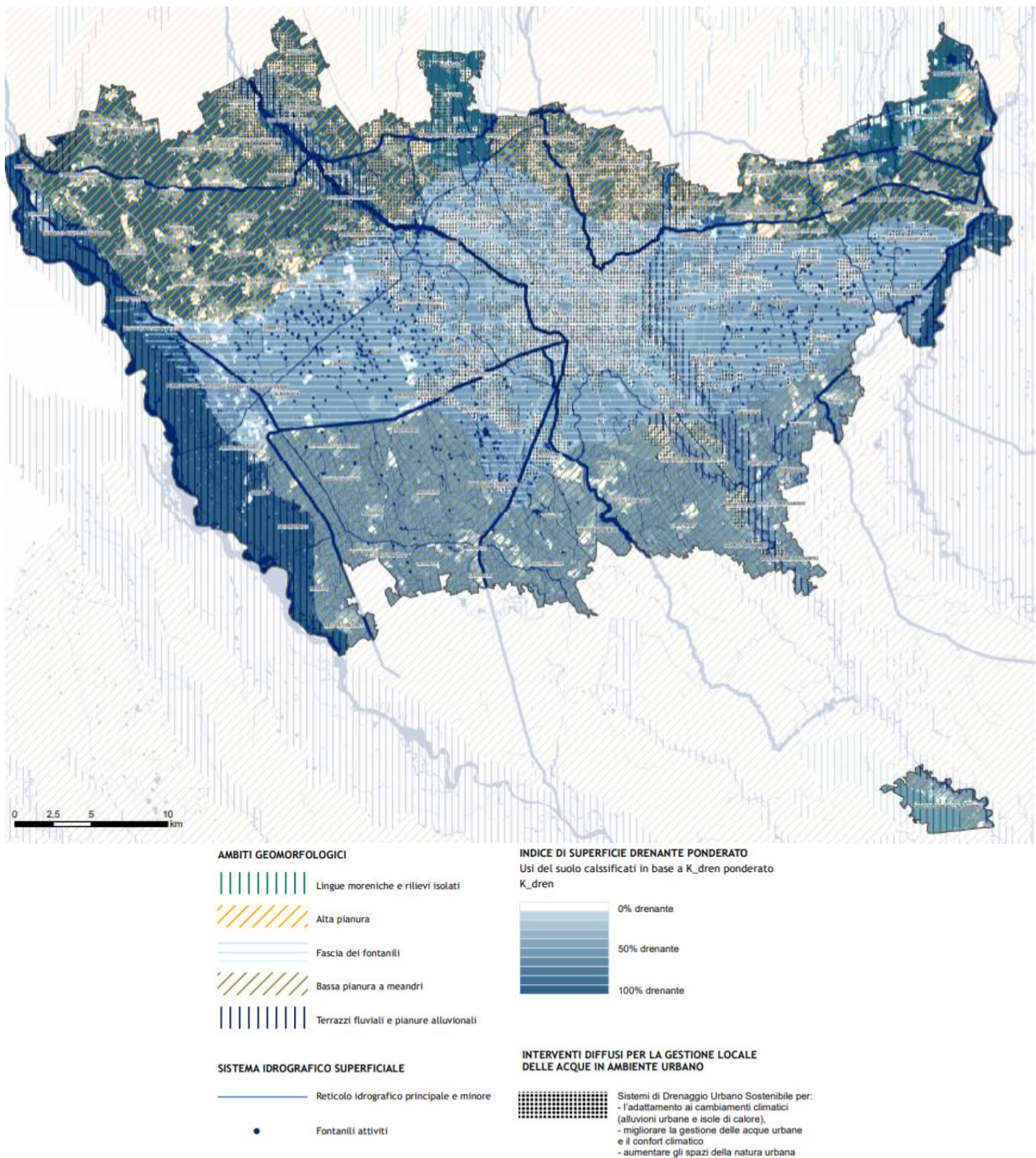
Figura 23. Laminazione degli eventi meteorici: schema e legenda
